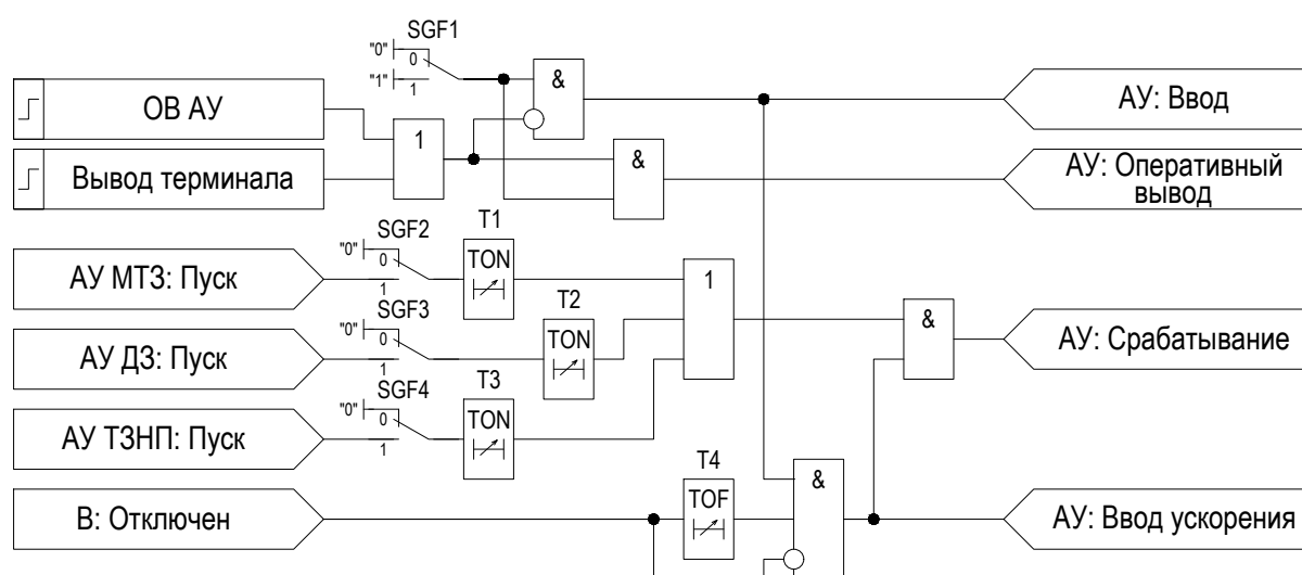
Рисунок 2.13 – Функциональная схема «АУ»
