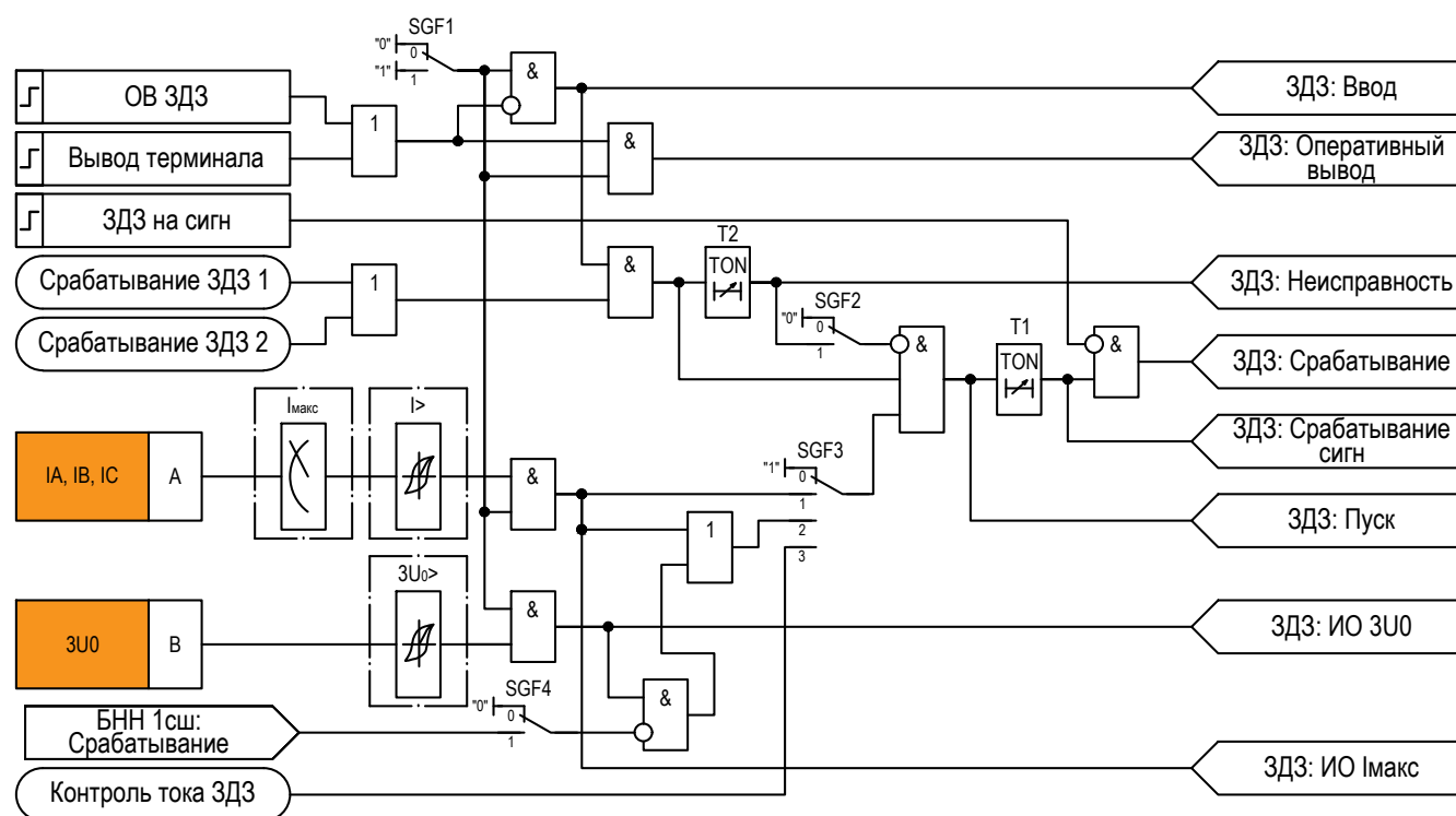
Рисунок 2.25 – Функциональная схема «ЗДЗ»
